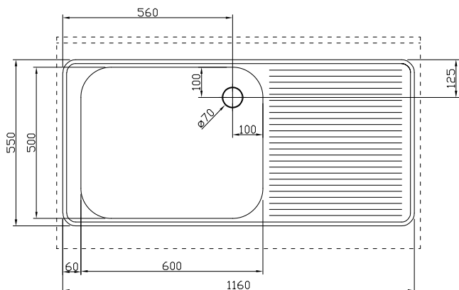
Planta
